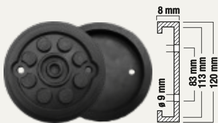
Para elevadores compatible con Maha, Euroli
