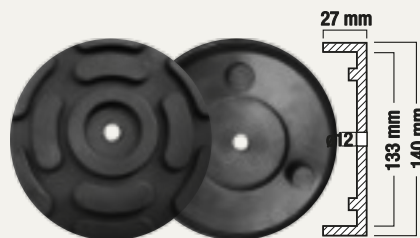
Taco de goma 20 140 mm para elevador de taller OM
