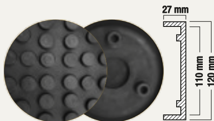
Taco de goma 18 de 120 mm para Ravaglioli...
